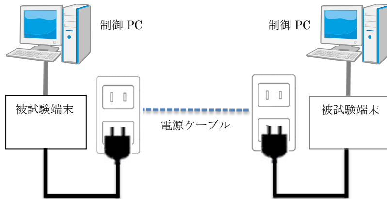
図 4-2-1 物理的接続イメージ
